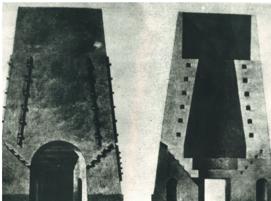
Pierwszy w Europie wielki piec hutniczy, opalany koksem z 1796 roku, konstrukcji Johna Baildona. (Fotografia ze zbiorów M. Grzelewskiej)
