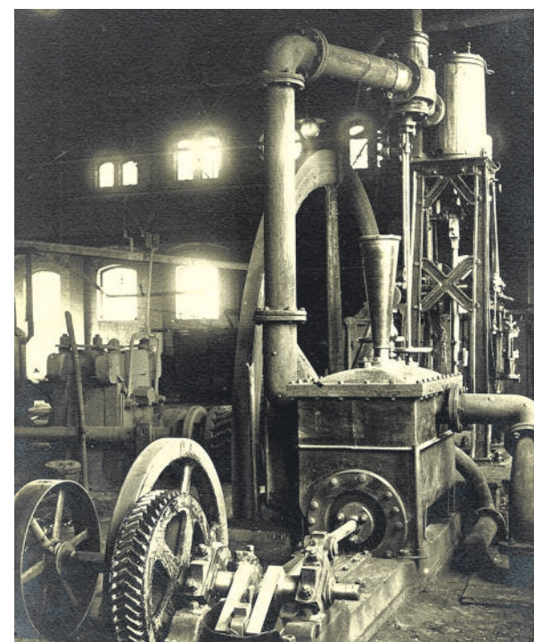
Maszyna parowa w hucie „Hermiona”, Łąbędy 1904 r. (Ze zbiorów Muzeum w Gliwicach).
